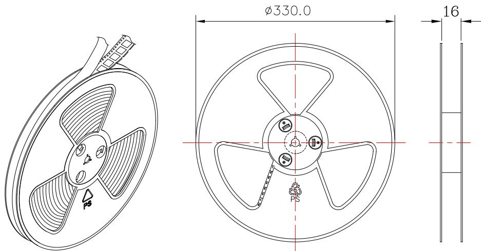
1 Reel : 2500PCS
